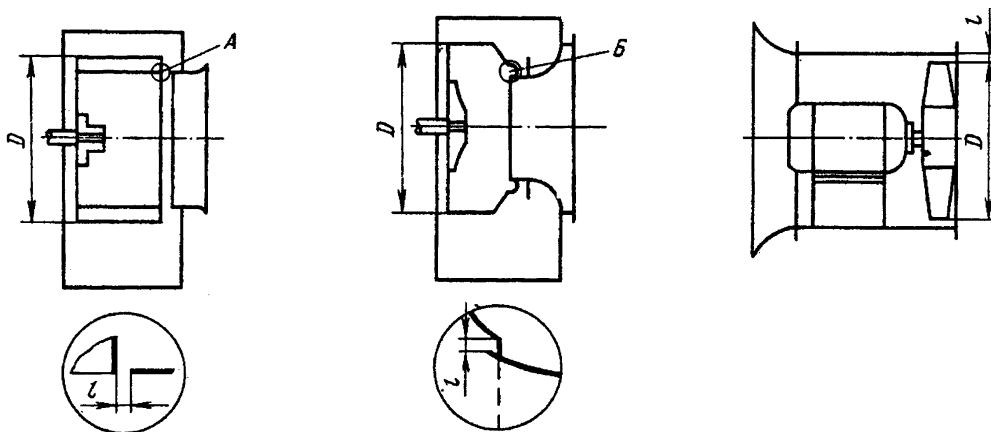
Рис. 2. Схемы зазоров вентиляторов: а - радиальных типа В.Ц14-46; б - радиальных типа В.Ц4-70; в - осевых ( t = 0,5-1,0\%D )
